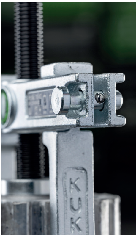
Gefederte Kugel sichert den Stift vor dem Herausrutschen
