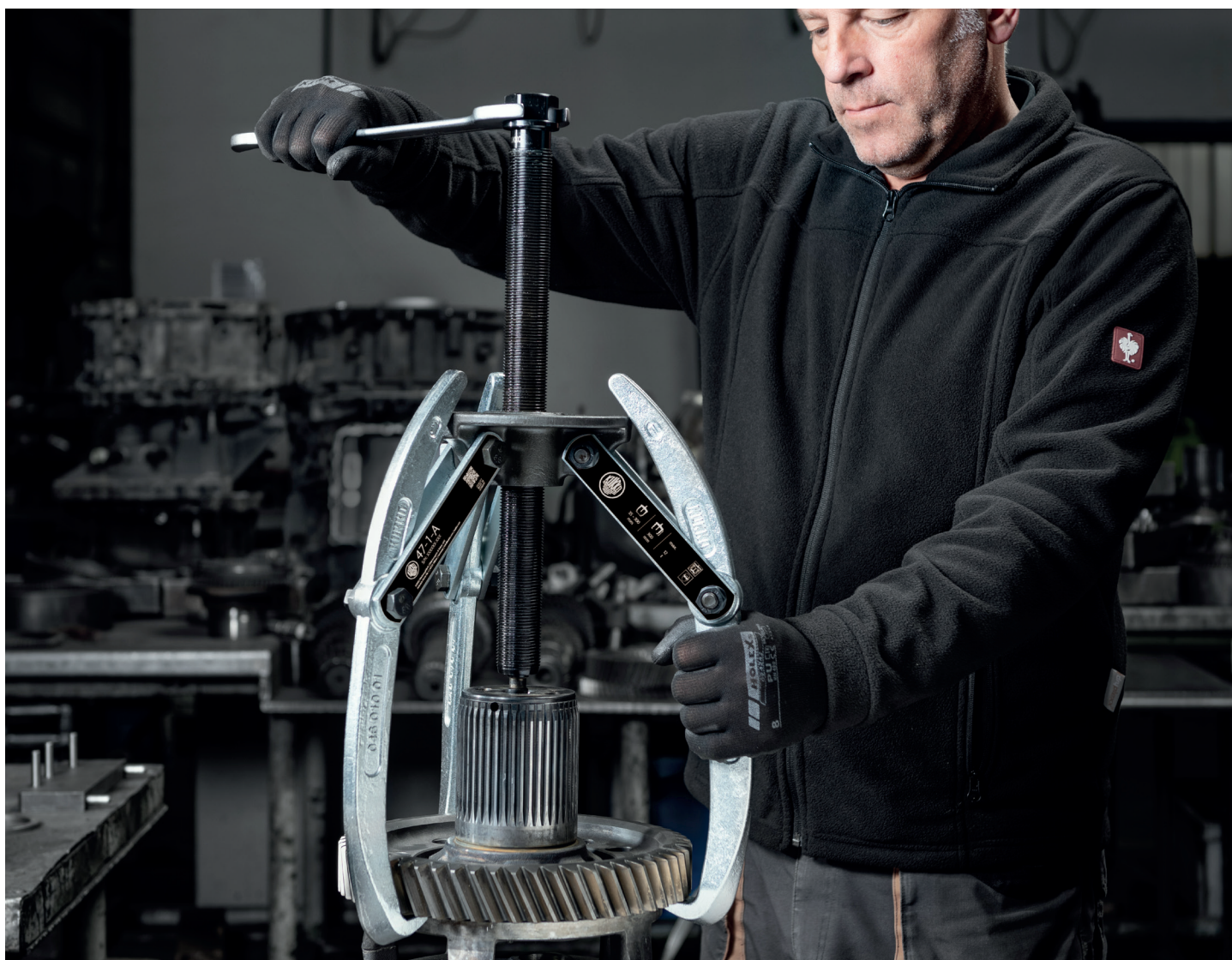
Abziehen eines Zahnrades mit dem 47-1-A
