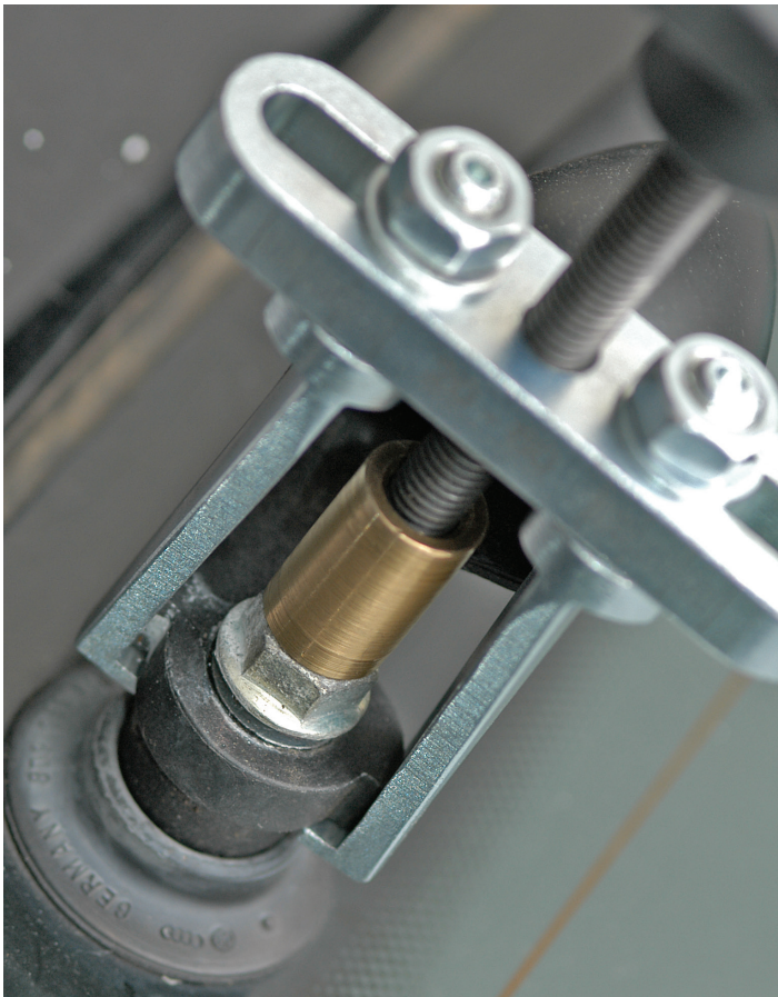
Abziehen eines Scheibenwischerarms mit dem 128-F-SW
